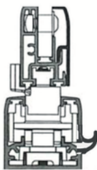
Geïntegreerde waterafvoer
